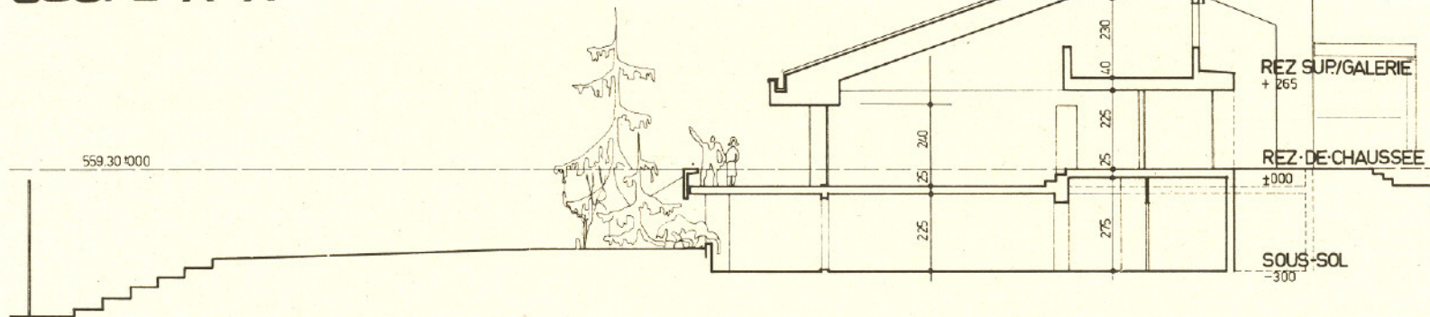
COUPE A-A
