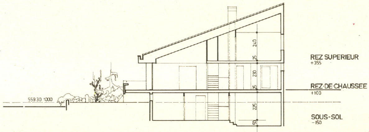
COUPE A-A
